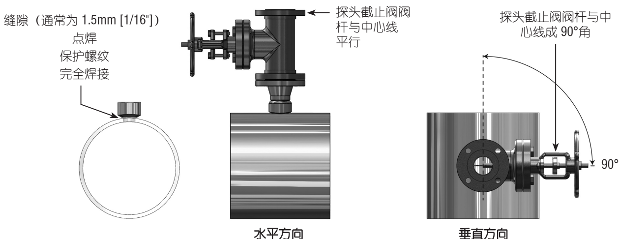
图 5. 探头截止阀
