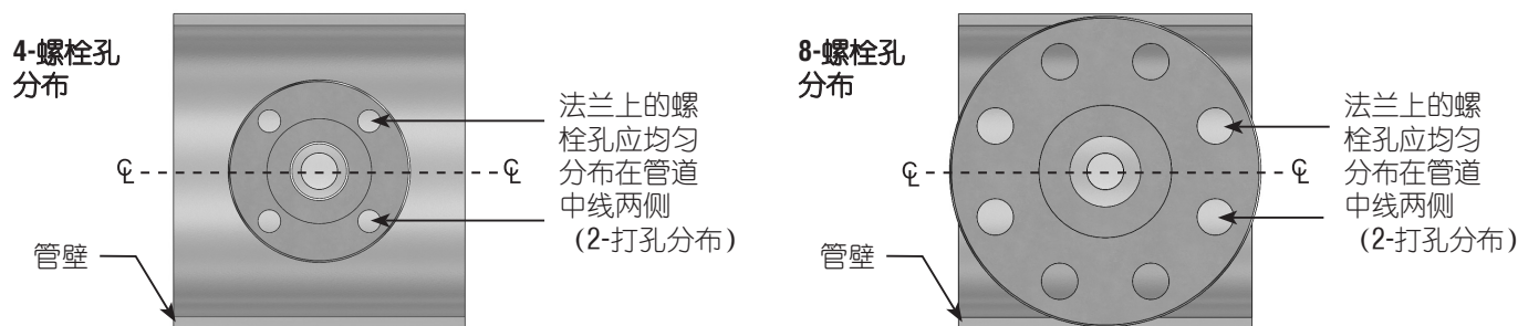
图 4. 法兰方向
